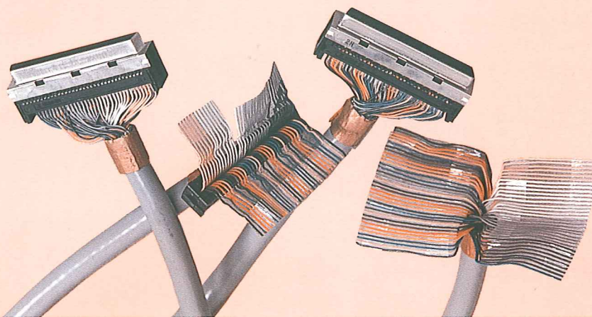
1.27ピッチ 細径1列平型(GH-4)
