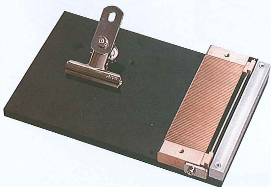
1.27ピッチ レギュラーサイズ用平型(GH-3)
